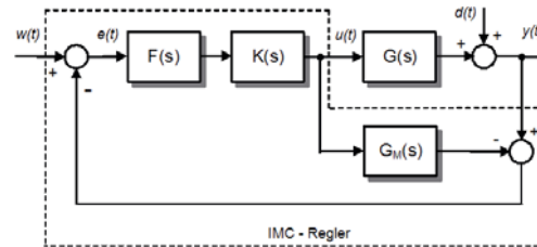
Beispiel: Reglerstruktur
