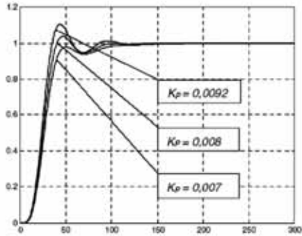
Beispiel: Einschwingvorgänge
