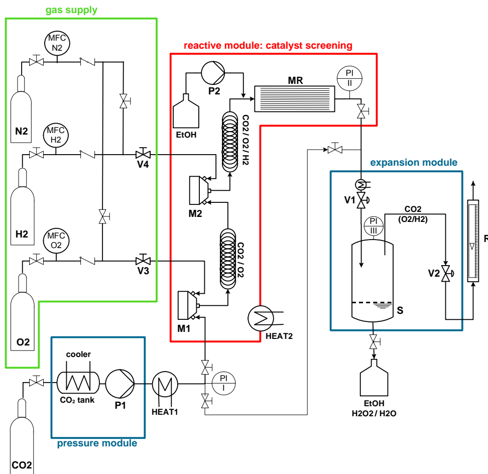
Abb. 1: Fließschema des Laborsystems zur kontinuierlichen H_2O_2 -Direktsynthese
