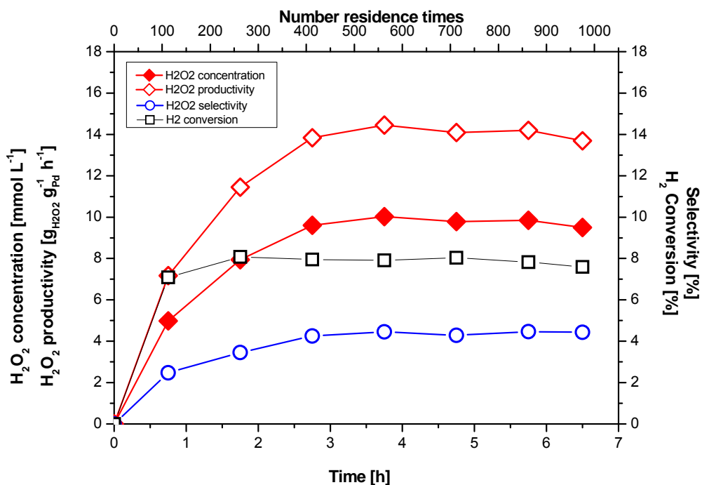
Abb. 27: Typischer Verlauf der kontinuierlichen Reaktion in \text{CO}_2/\text{EtOH} für einen 5%Pd- \text{TiO}_2 Katalysator. Reaktionsbedingungen: T_{\text{sys}} = 27^\circ\text{C} ; P_{\text{sys}} = 13.5\text{ MPa} ; F(\text{H}_2) = 1.3 \cdot 10^{-2}\text{ mol min}^{-1} ; \text{H}_2/\text{O}_2/\text{CO}_2 = 17/34/49\text{ mol } \% ; F_{\text{CO}_2} = 40\text{ Ln min}^{-1} ; F_{\text{EtOH}} = 4.8\text{ mL min}^{-1} ; m_{\text{Pd}} = 6.7\text{ mg} .
